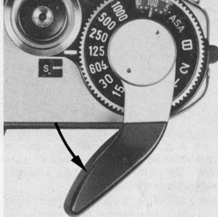
Levier de blocage du déclencheur
